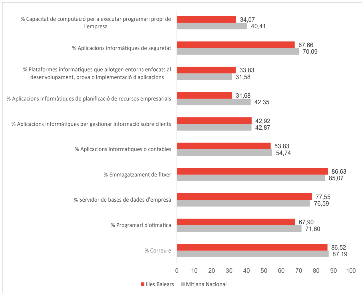
Gràfic 18: Resum Cloud Computing (%). Illes Balears i mitjana estatal
